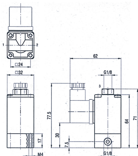
Ingombro / Dimensions
