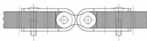
GIUNZIONI SNODATE DISPONIBILI "Z" ARTICULATED CONNECTOR AVAILABLE TYPE "Z"
